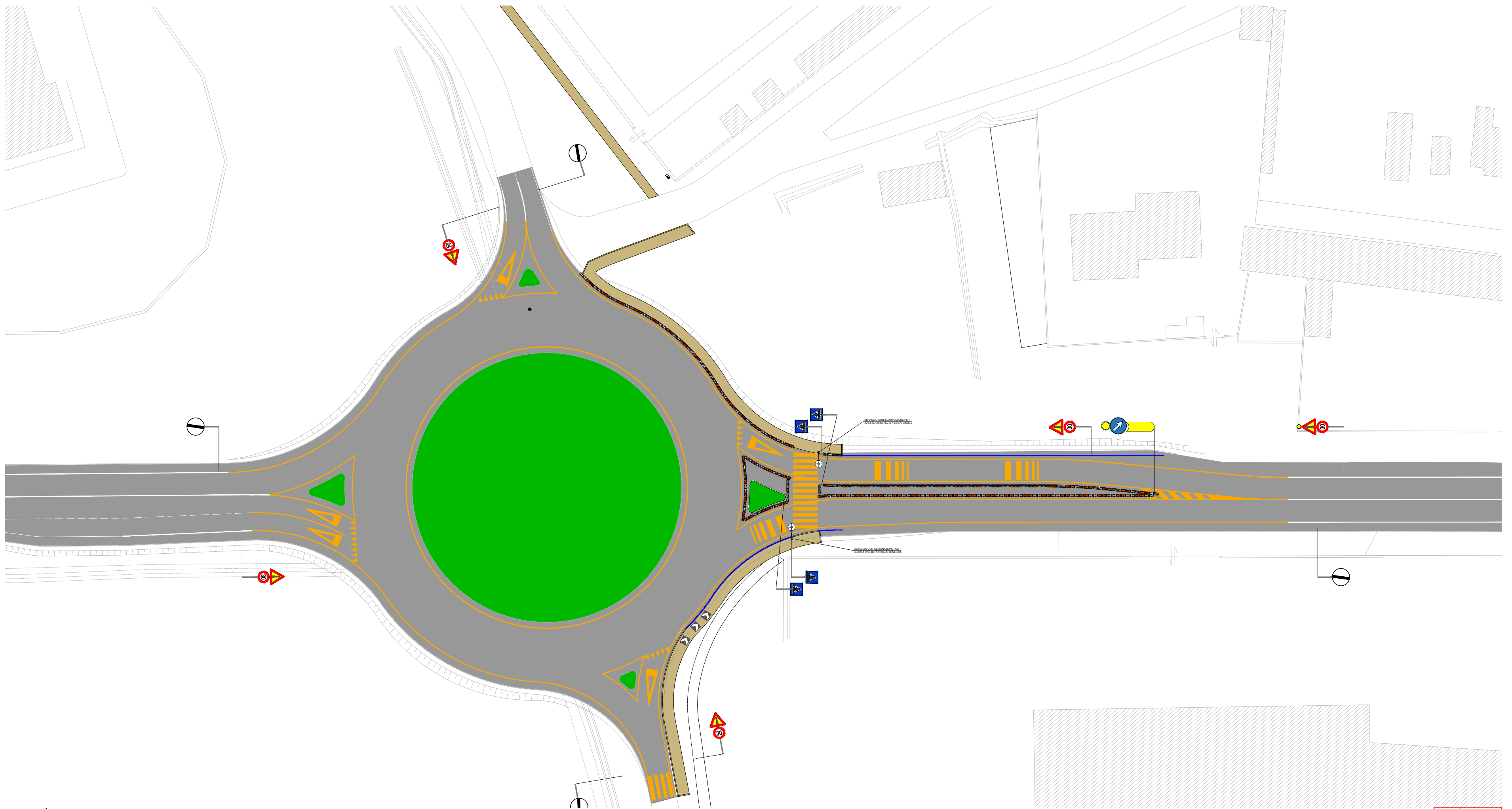
Ipotesi di attraversamento pedonale sulla SP11 a Vittuone
