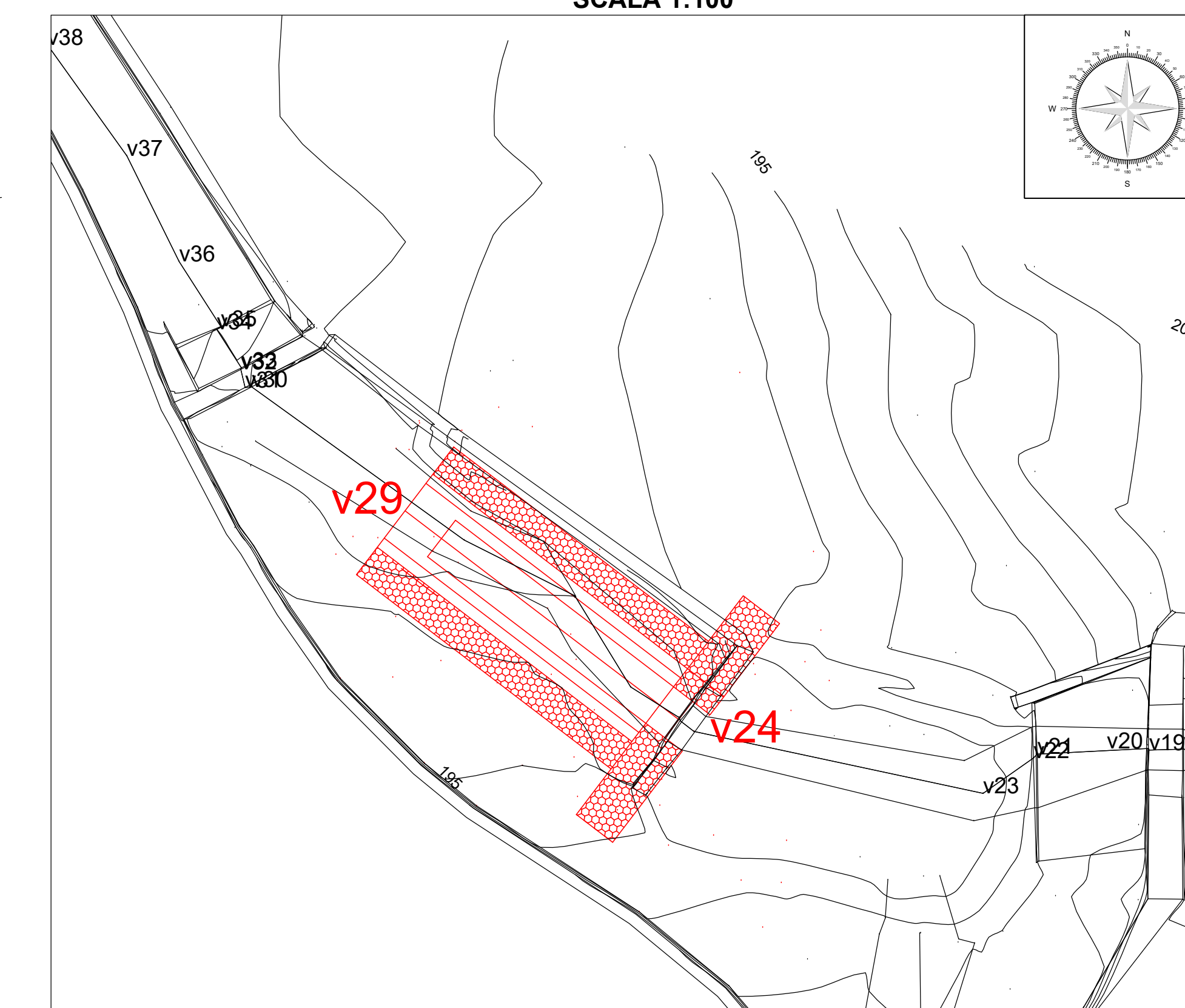
INQUADRAMENTO GENERALE SCALA 1:100
