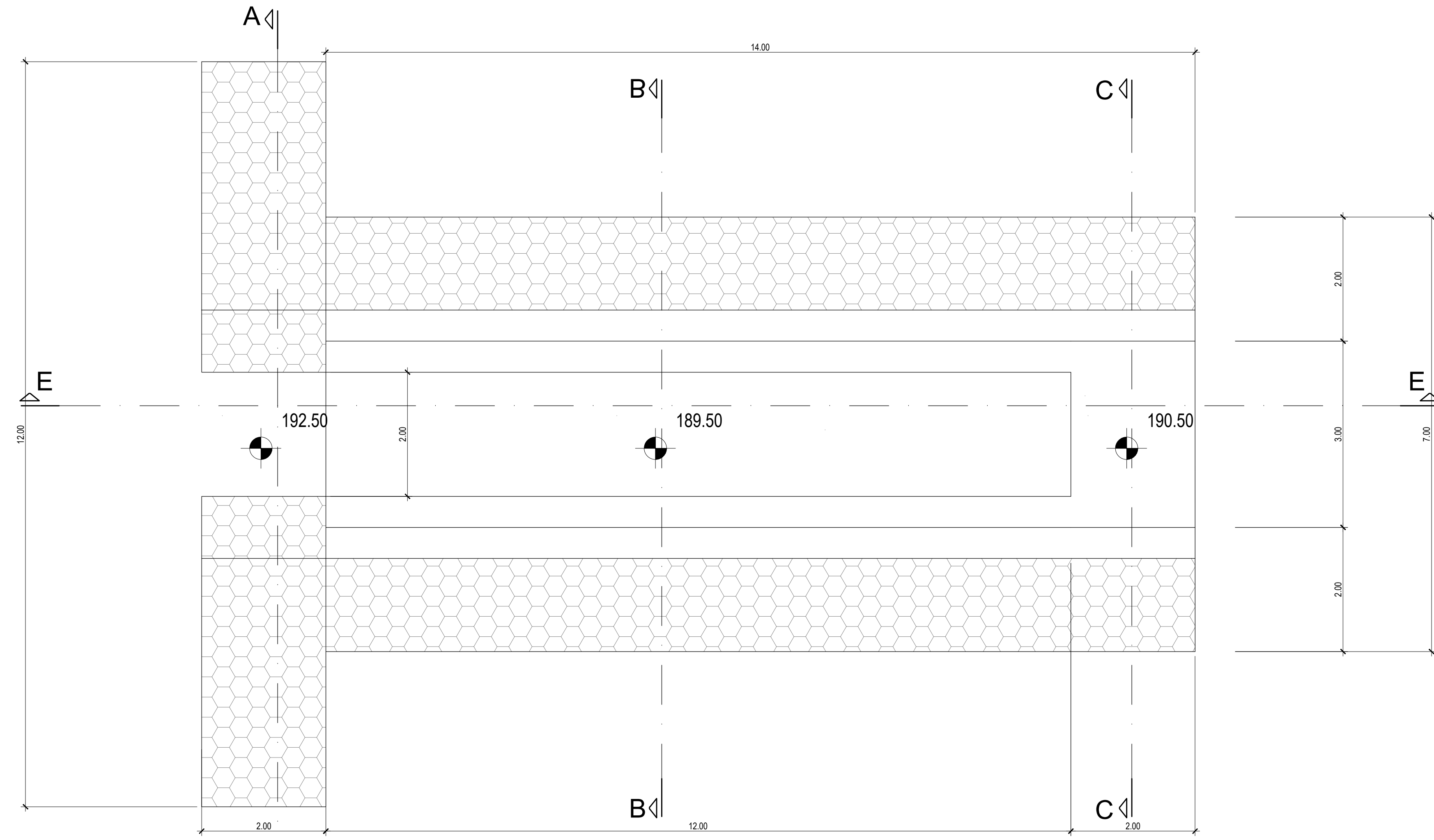
PIANTA DELLA BRIGLIA SCALA 1:50
