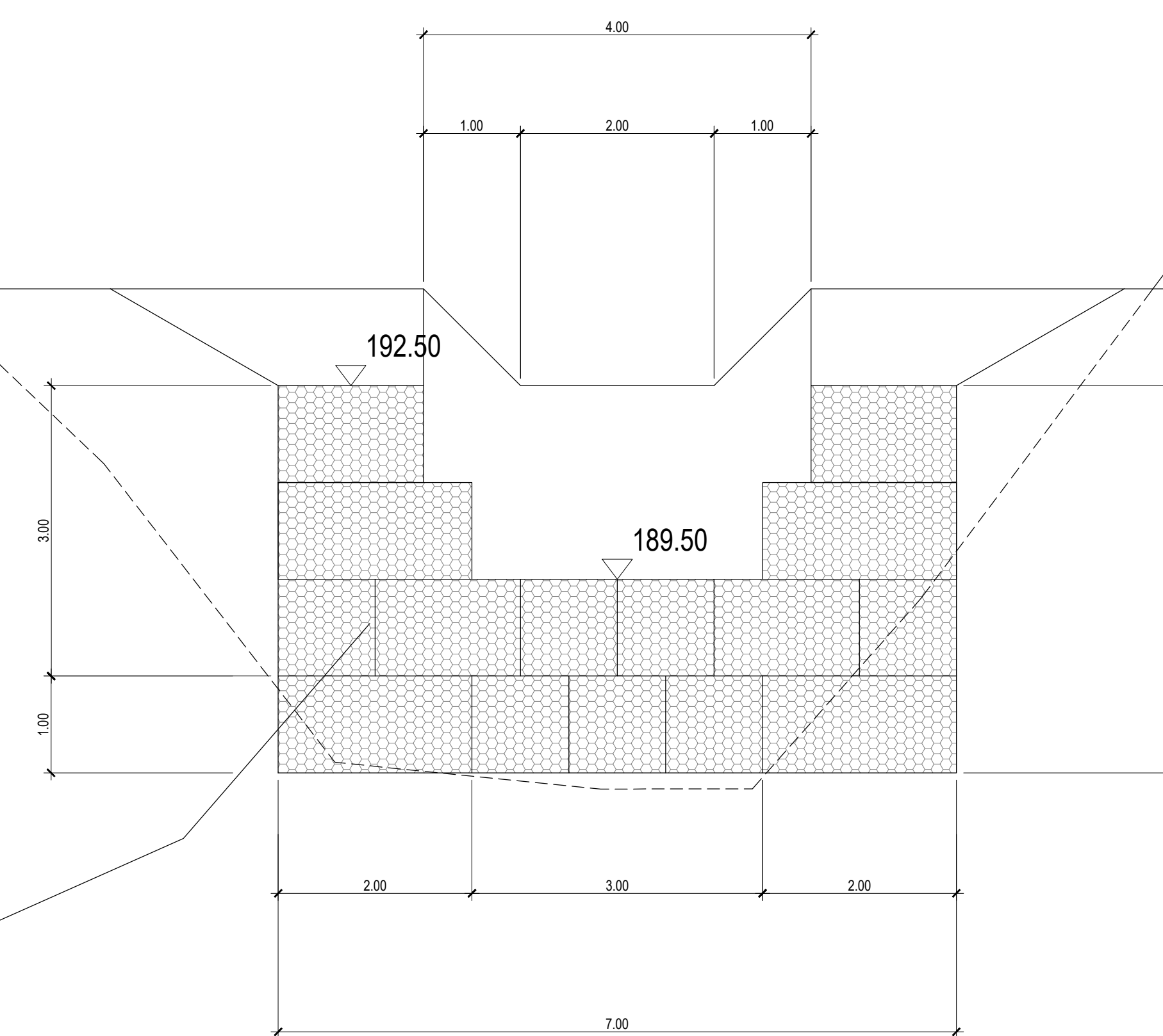
SEZIONE C-C SCALA 1:50
